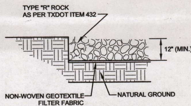
ROCK RIPRAP DETAIL N.T.S.
